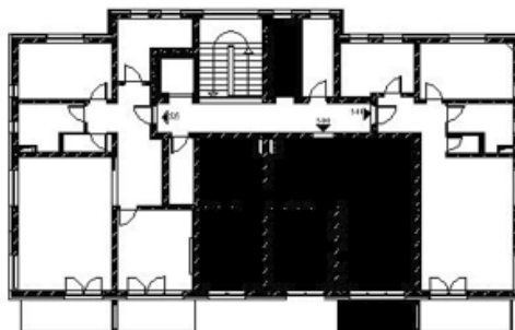
Blok A - 2. nadstropje
