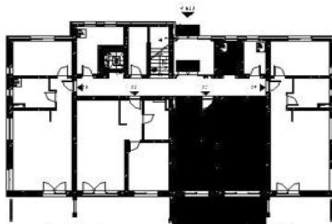
Blok A - Pritličje
