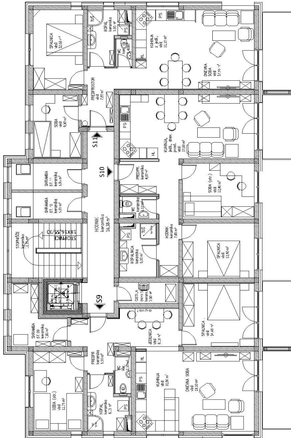
TLORIS 2. NADSTROPJA - OBJEKT A
