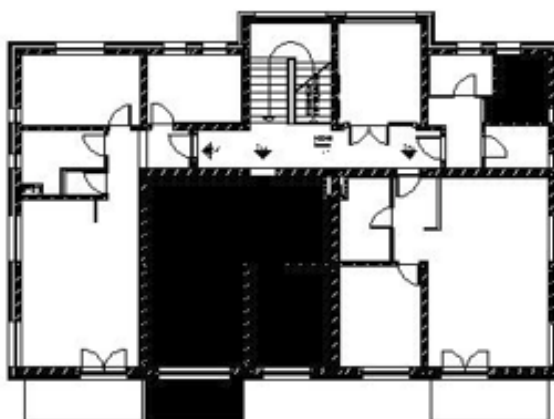
TIGRIS 1. NADSTROPJE - ČRTEŽ B
